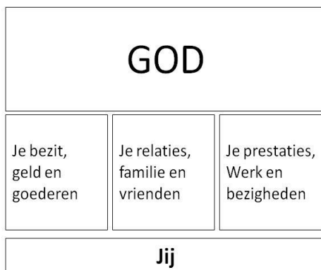
Schema 1.
